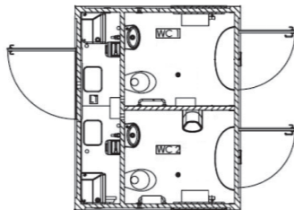
2.40 m x 2.96 m H 2.58 sanitaire double + local technique
