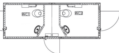
1.50 m x 4.00 m H 2.58 sanitaire double + local technique
