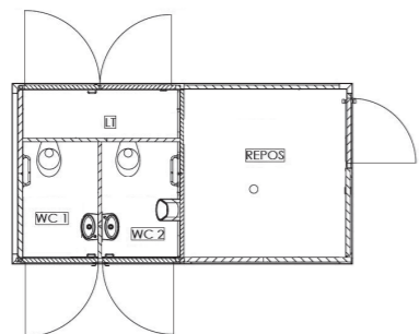
2.40 m x 4.50 m H 2.58 sanitaire double + repos + local technique
